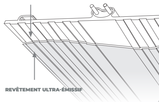
STRUCTURE MONOBLOC EN ALUMINIUM
