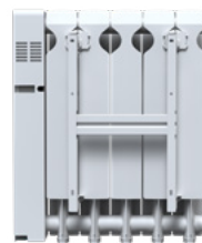
Fixation en H auto-gabarit, ce qui facilite le positionnement de l'appareil au mur sans prise de côtes.
