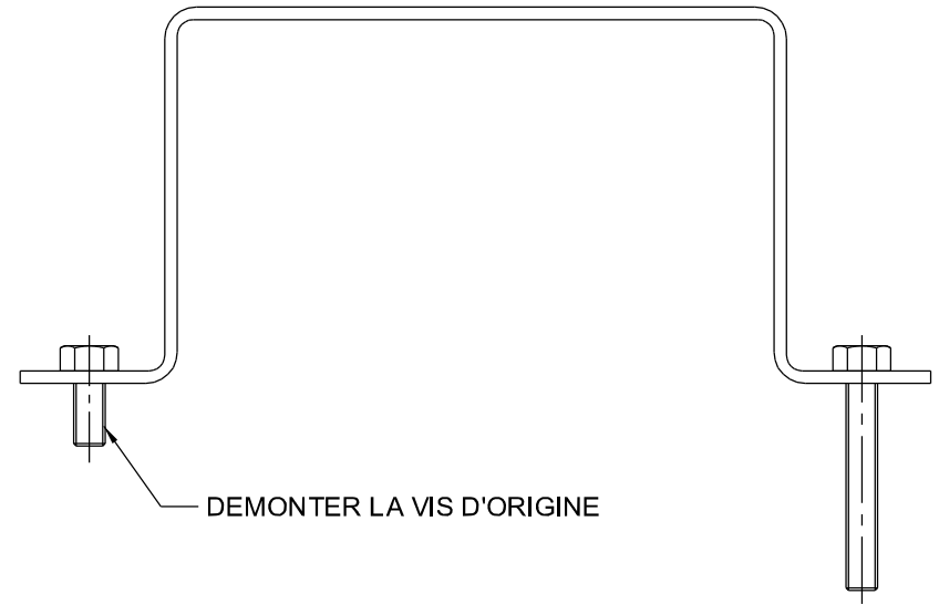
POIGNEE PULSATOIRE 32/40 D'ORIGINE
