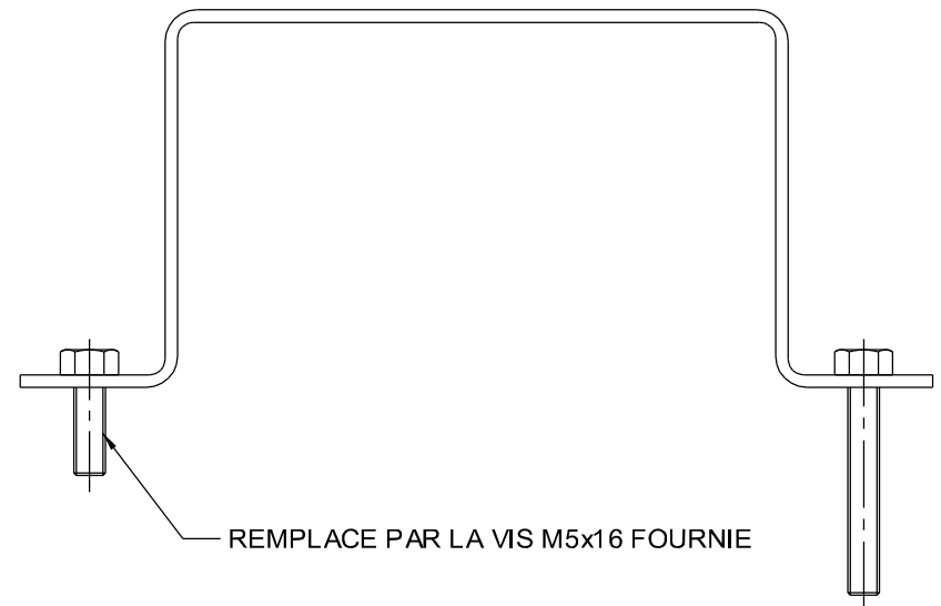
POIGNEE PULSATOIRE 32/40 MODIFIEE
