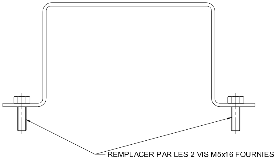
POIGNEE PULSATOIRE 20 MODIFIEE
