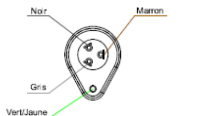
Bornier compresseur version 1
