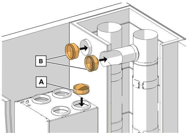
A - Clapet antiretour B - Clapet coupe-feu (non fourni)
