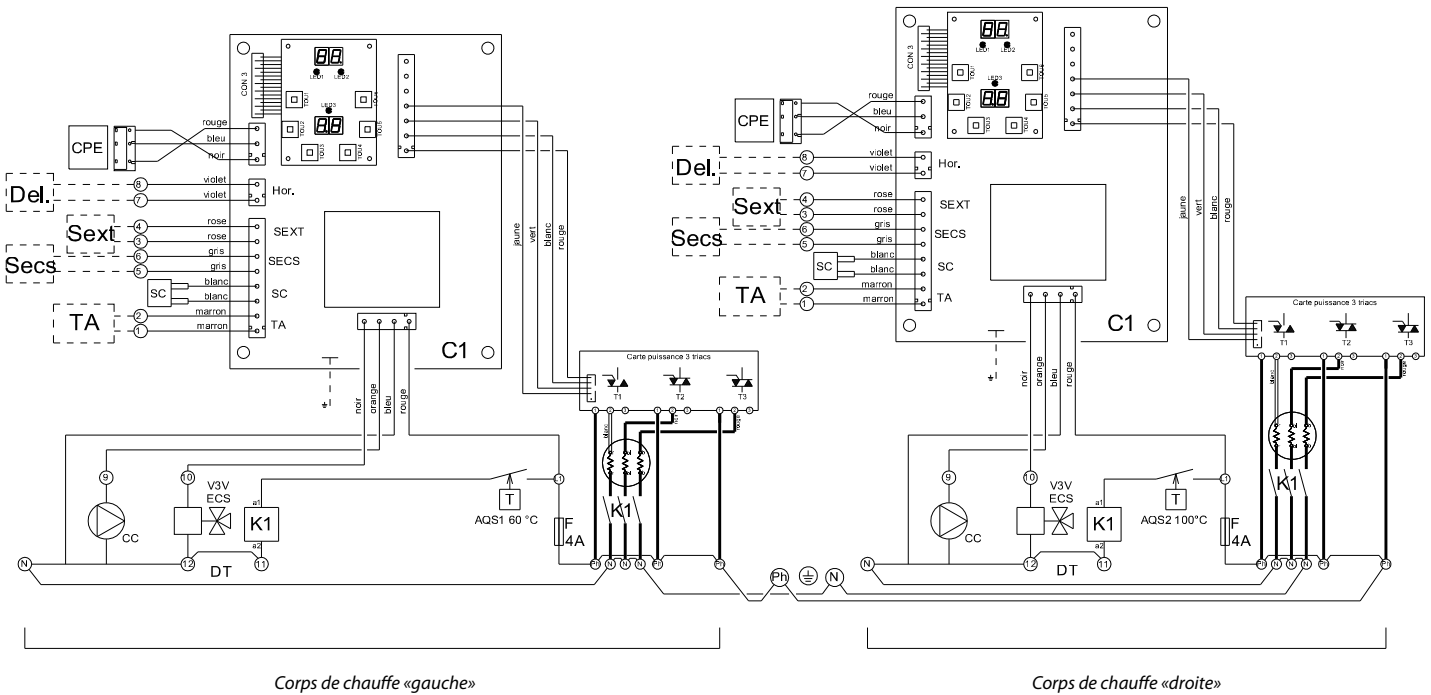
Corps de chauffe «gauche»
