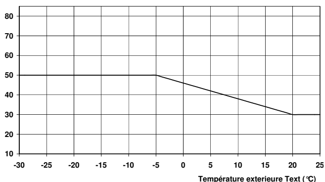
Température de consigne départ chaudière TC (°C)
