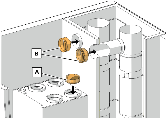
A. Clapet antiretour Ø 160 B. Clapet coupe-feu (non fourni)
